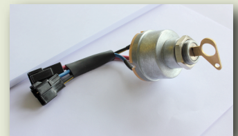
GE's Item Code : 765-05 Starter Switch
